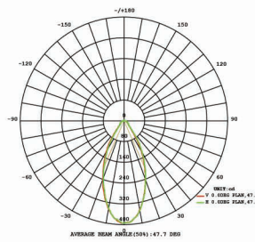
5.5W Module
